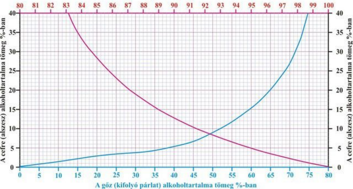
A cefre (alszesz) forráspontja Celsius fokban
