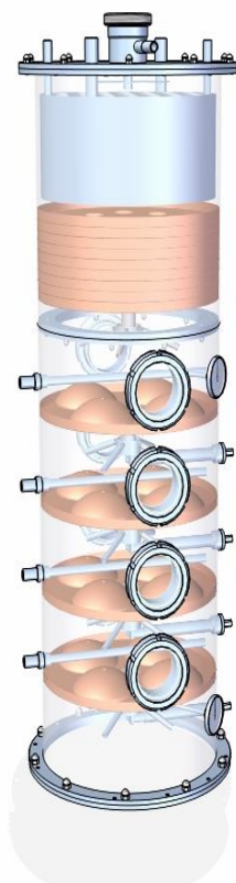
7. ábra: Hagyó féle rektifikáló oszlop (forrás: Hagyó kft., Miskolc)
