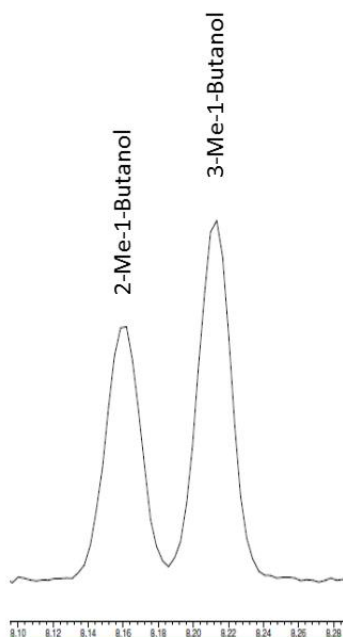
9. ábra: Amilalkoholok elválasztása CP-WAX 57 CB oszloppal
